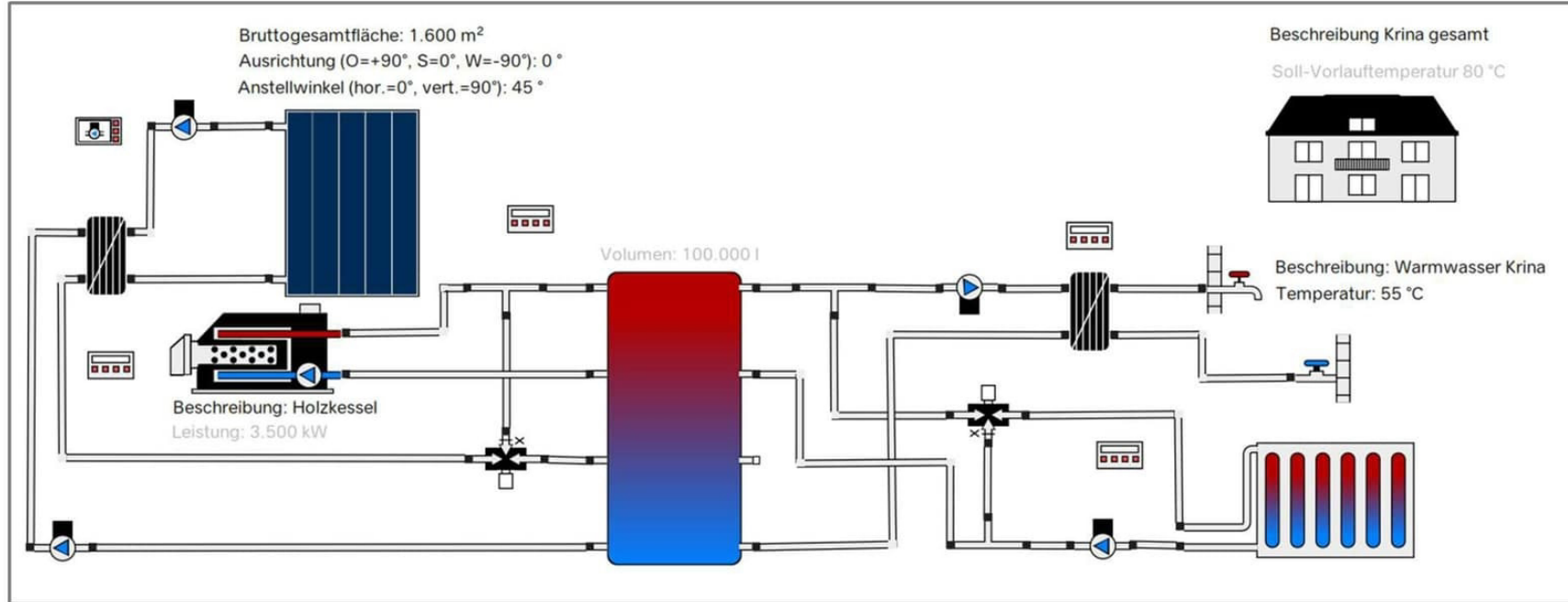
Abbildung 46 | Anlagenschema der Polysun-Simulation für Krina, Variante 2 mit Solarthermie-Anlage
