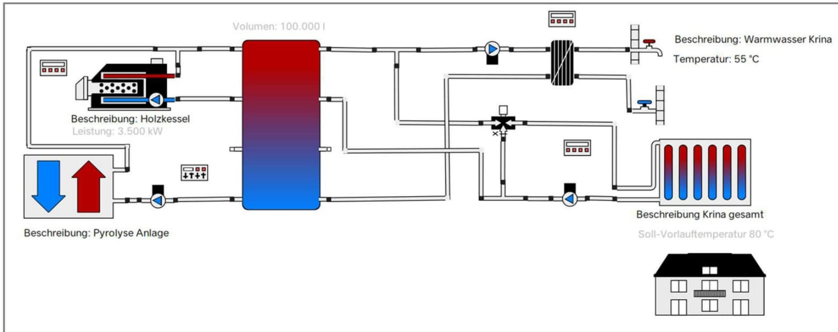
Abbildung 45 | Anlagenschema der Polysun-Simulation für Krina, Variante mit Pyrolyse-Anlage
