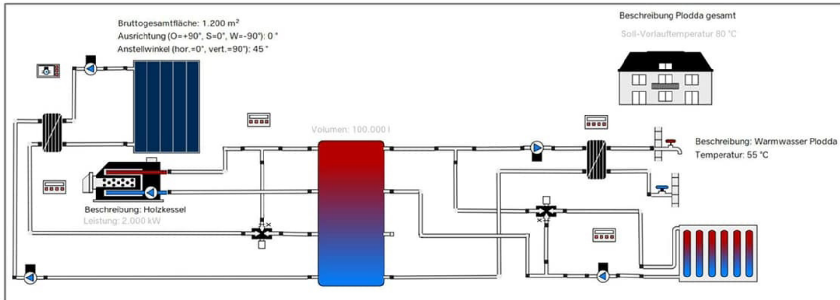
Abbildung 40 | Anlagenschema der Polysun-Simulation für Plodda
